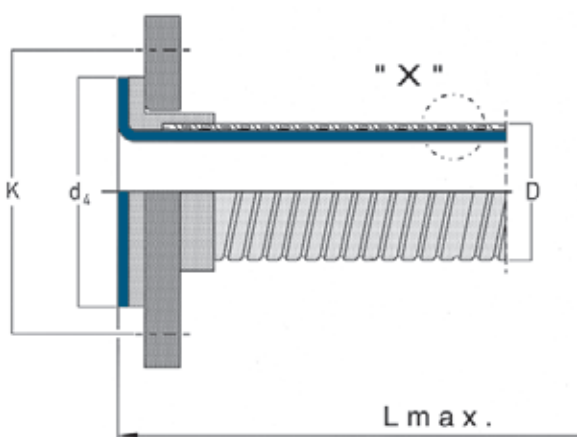
Detail „X“
